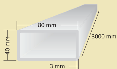
Mât de 3 m, section 80 x 40 mm
