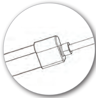
Option Entrée n°1 Sortie longitudinale du câble d'alimentation du FLEXIMAT
