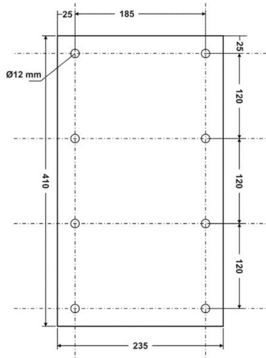
Pied de fixation
