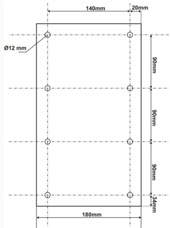
Pied de fixation
