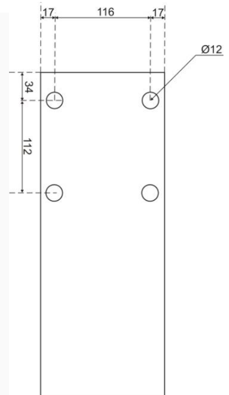
Pied de fixation (Dim en mm)
