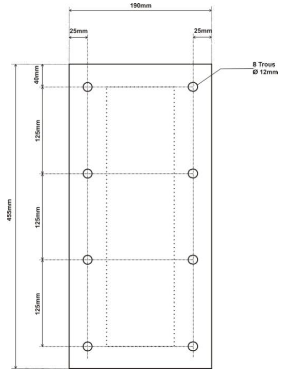
Pied de fixation
